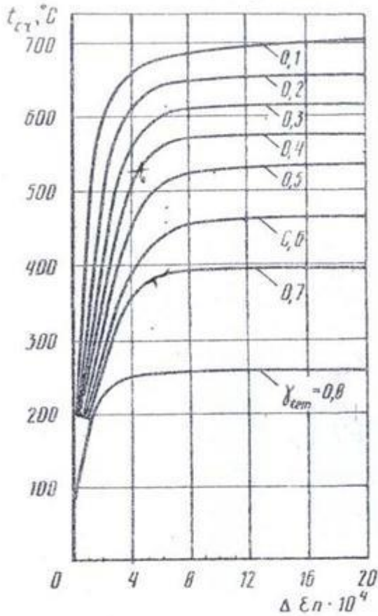
Кривые критических температур, вызывающих потерю устойчивости сжатых стальных стержней: \Delta \epsilon_n – критическая разность краевых деформаций ползучести; \gamma_{сеп} – степень нагружения стержня
