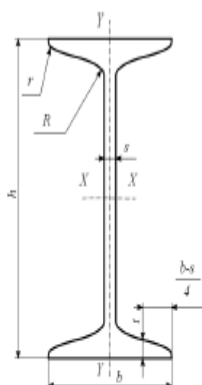
Приложение 6. Двутавры стальные горячекатаные. ГОСТ 8239-89 (фрагмент)
